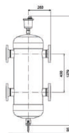
SEPARADOR HIDRAULICO
